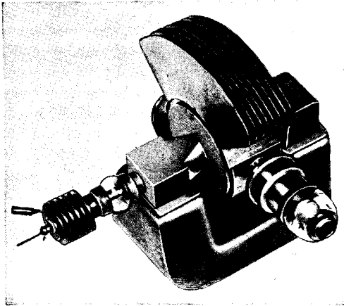
FIG. 19-7.—CM16B magnetron.
